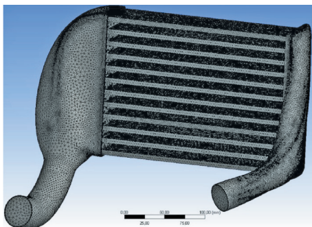
Рис. 3. Твёрдотельная модель расчетной области ОНВ варианта № 5 с расчетной сеткой
