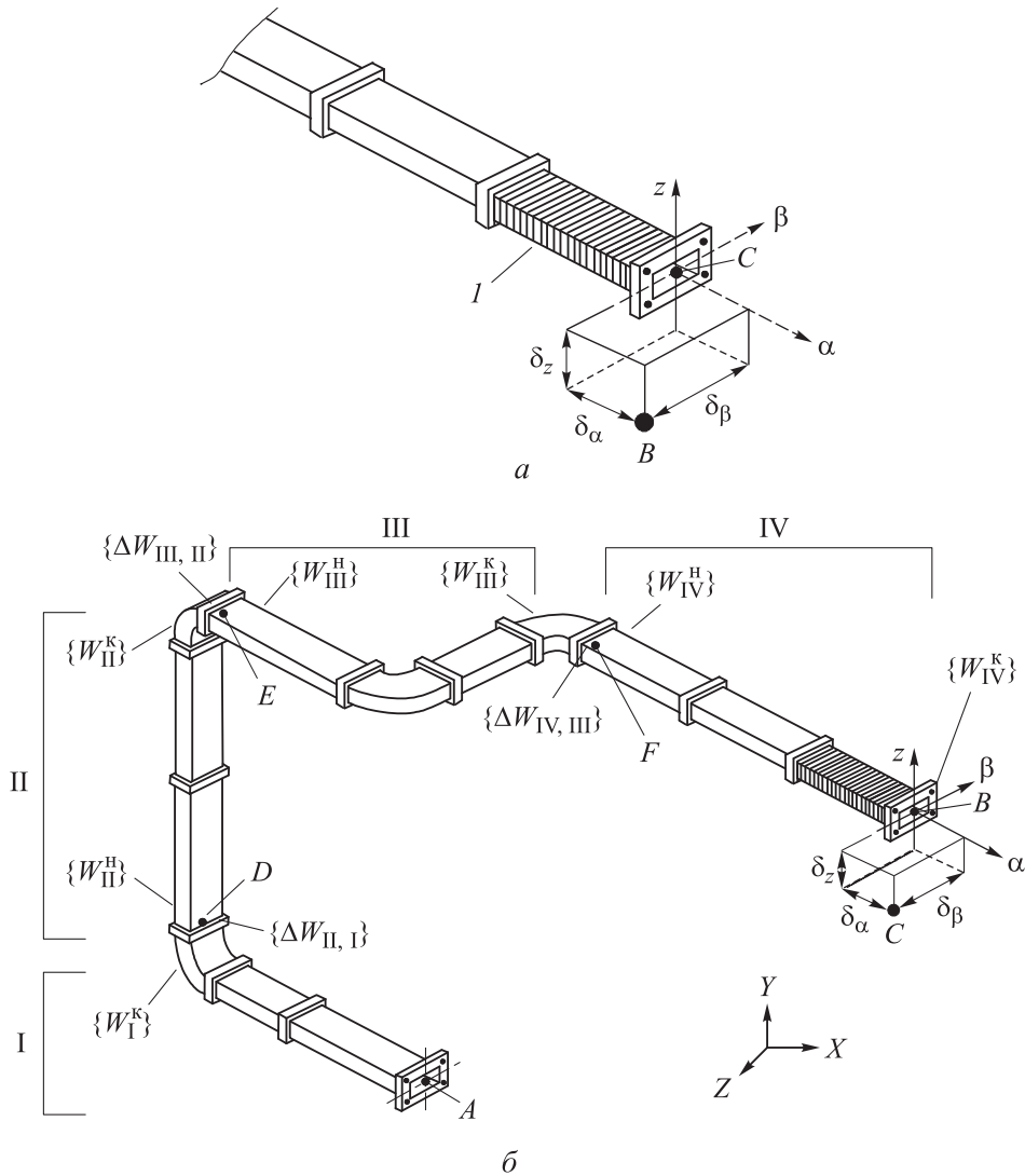
Рис. 3. Отклонения характерных точек участка волновода от требуемых положений: I — гибкая секция; \{\Delta W_{II,I}\} , \{\Delta W_{III,II}\} и \{\Delta W_{IV,III}\} — вектор отклонения соответственно участка II относительно участка I, участка III относительно участка II и участка IV относительно участка III; \{W_I^K\} — вектор перемещения в конце участка I; \{W_{II}^H\} , \{W_{II}^K\} и \{W_{III}^H\} , \{W_{III}^K\} — векторы перемещения в начале и конце участка II и III соответственно; \delta_\alpha , \delta_\beta и \delta_z — смещение конечной точки B по осям \alpha , \beta и z соответственно; A, D, E и F — точки, определяющие границы участков I, II, III и IV соответственно
