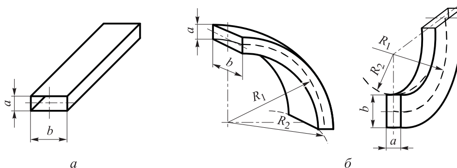
Рис. 1. Схемы прямого (а) и криволинейного (б) элементов ВРС: R_1, R_2 — радиусы кривизны элементов
